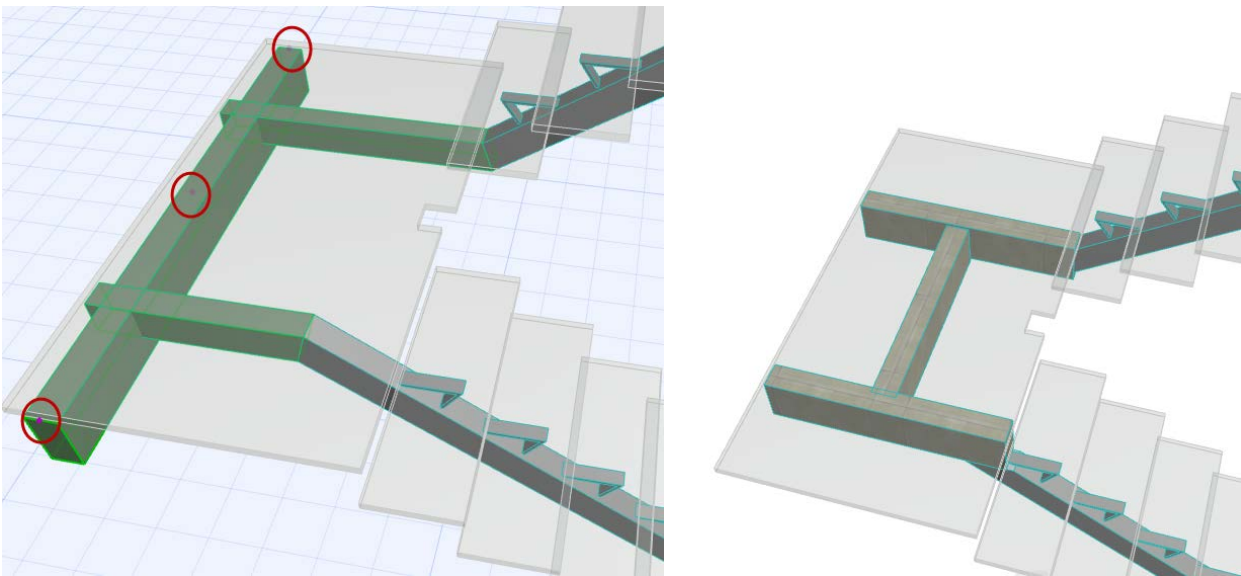
Modifier crémaillère secondaire graphiquement en mode d'édition
