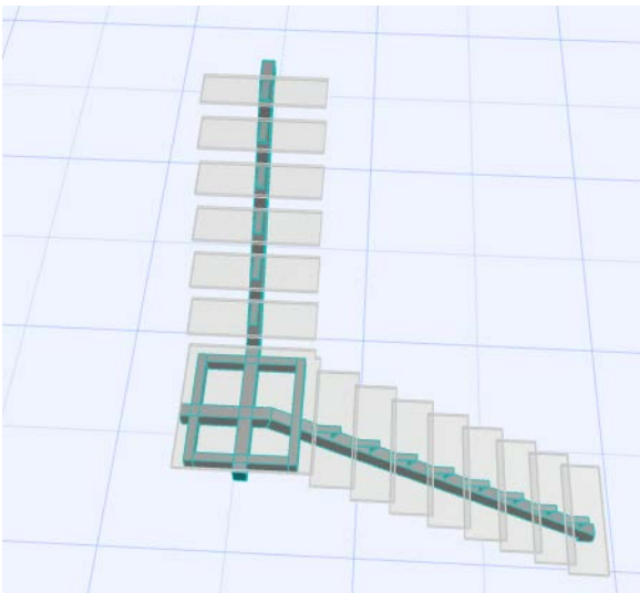
Paliers avec crémaillères primaires et secondaires
